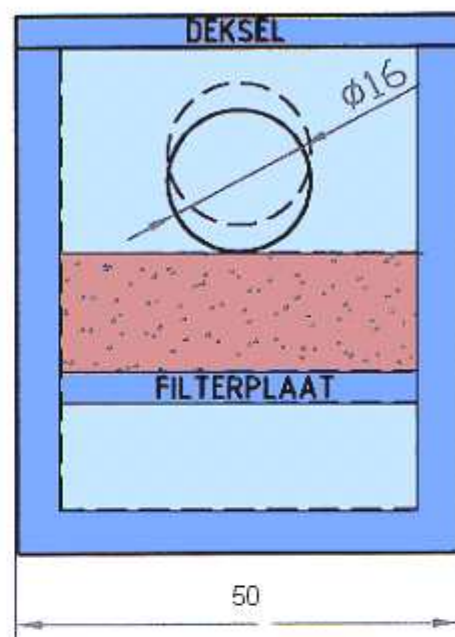
LINKERAANZICHT
