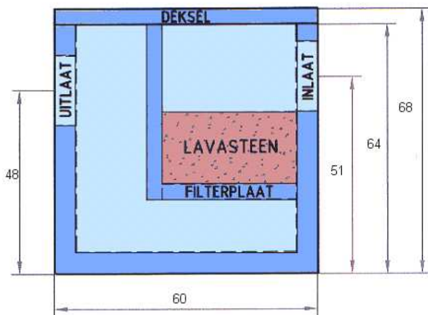
VOORAANZICHT
